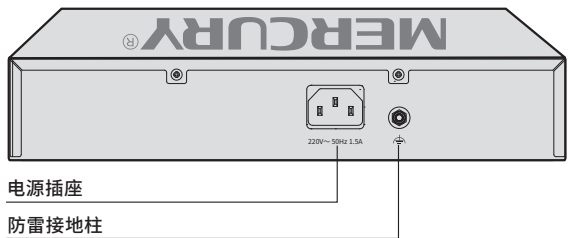
图 2-5 SE109P 后面板示意图
