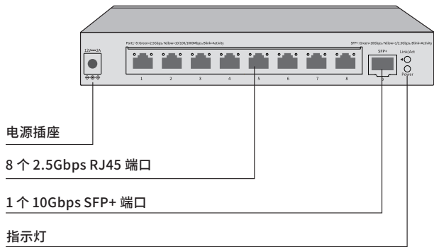
图2-4 SE109后面板示意图
