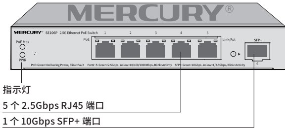
图 2-3 SE106P 前面板示意图
