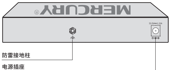
图 2-6 SE106P 后面板示意图
