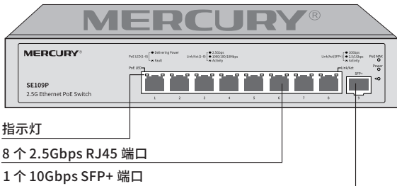
图 2-2 SE109P 前面板示意图
